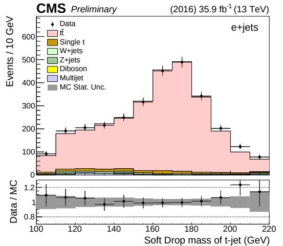
(f) 1t1b, e+jets
