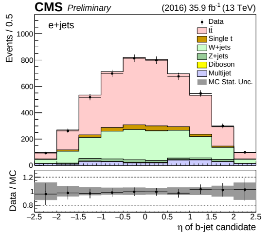
(d) 1t0b, e+jets
