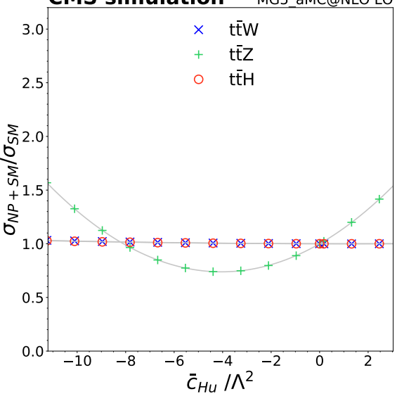
CMS simulation MG5_aMC@NLO LO
