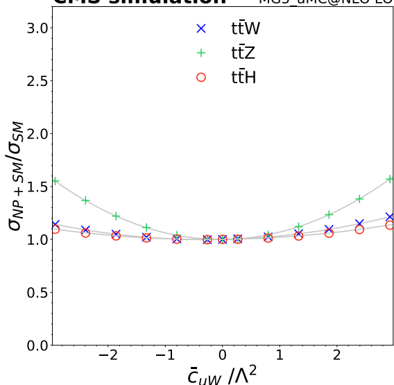
CMS simulation MG5_aMC@NLO LO
