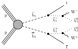
(d) T6ttWW
