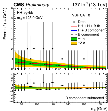
(d) VBF CAT 0
