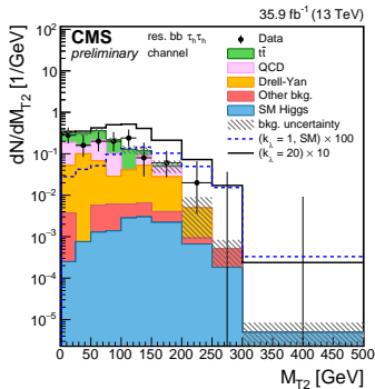
(d) resolved 2b0j - non-resonant
