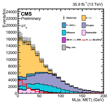
(d) M_T(e, E_T^{\text{miss}})
