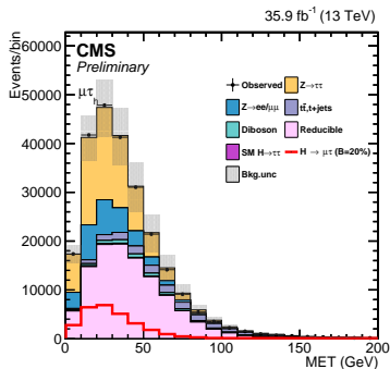
(d) E_T^{\text{miss}}
