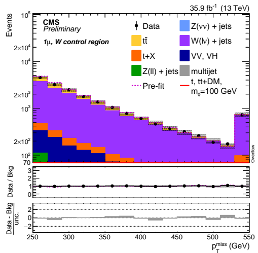
(d) AH1 \mu -W
