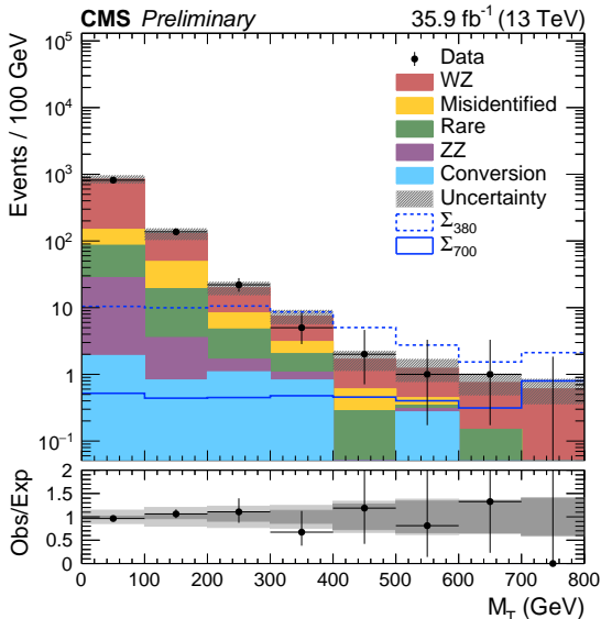
(a) M_T , L3OnZ
