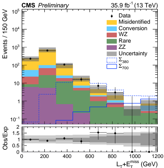
(d) L_T + E_T^{\text{miss}} , L3OSSF0
