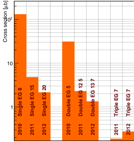
CMS \sqrt{s} = 7 or 8 TeV
