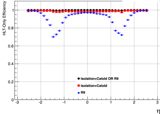
CMS 8 TeV
