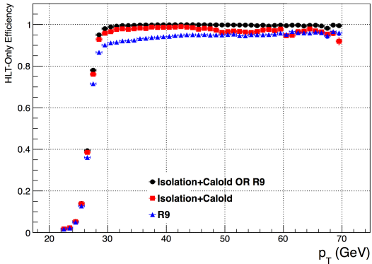
CMS 8 TeV
