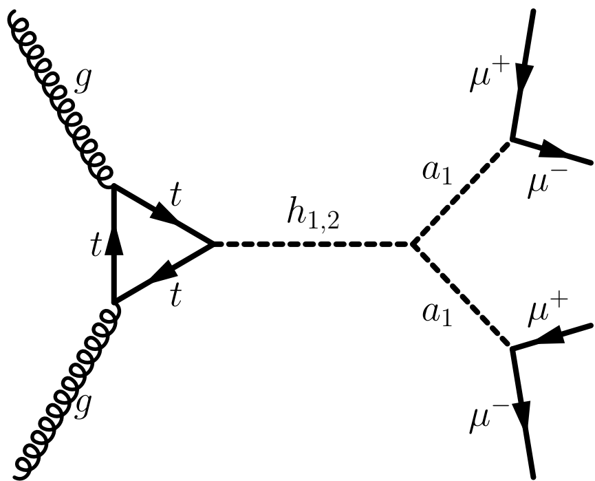
NMSSM
