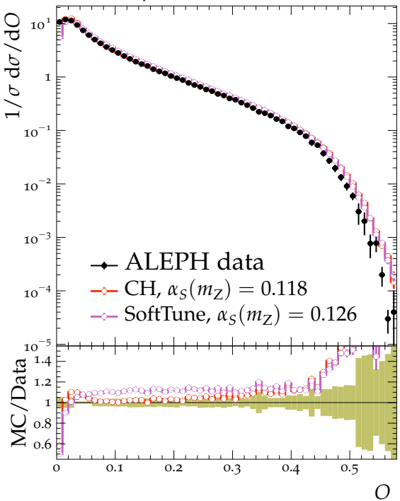
Oblateness, \sqrt{s} = 91.2 GeV
