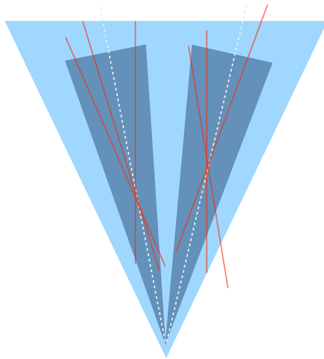
subjets
