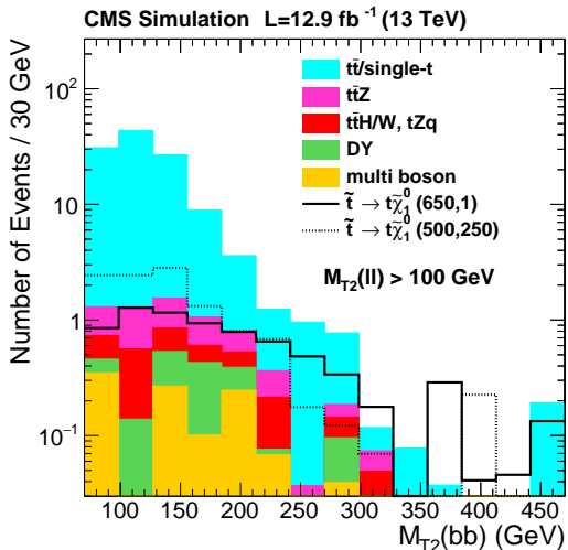
(b) M_{T_2}(bb)
