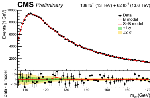
(d) ggF 4
