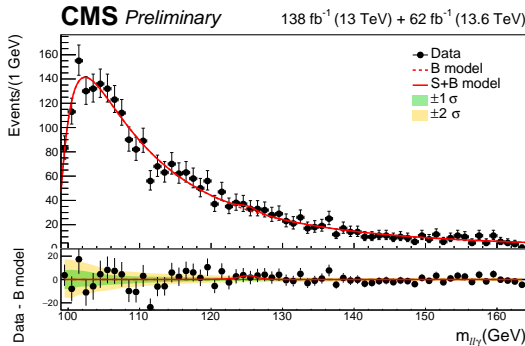
(b) ggF 2
