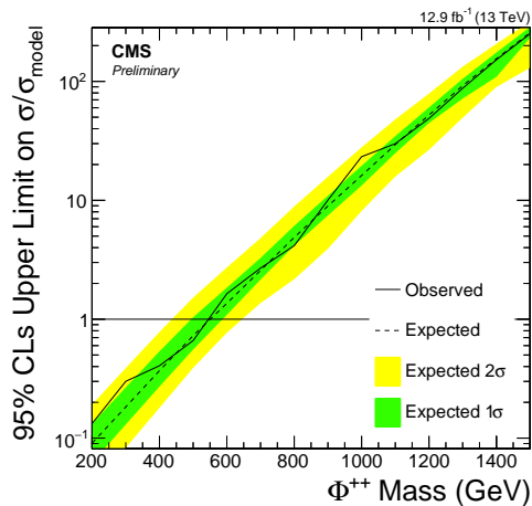
(d) 100% \tau\tau
