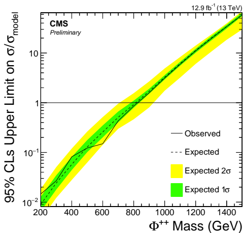
(d) 100% e\mu
