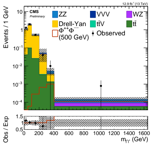
(d) l^\pm \tau^\pm l^\pm \tau^\pm
