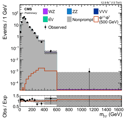
(d) l^\pm \tau^\pm \tau^\mp
