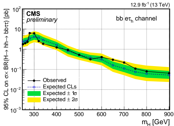
(b) bb e\tau_h
