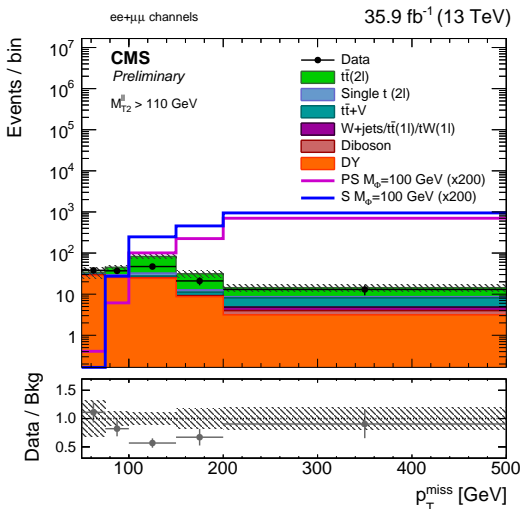
(d) high purity, ee + \mu\mu channels
