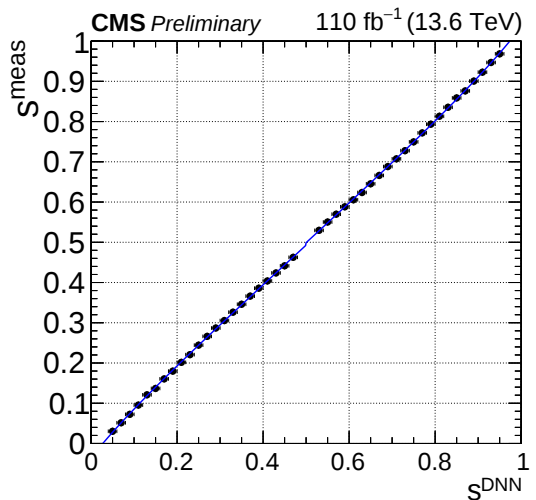
(d) SS tagger.
