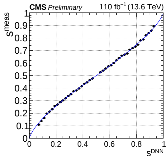
(c) OS-jet tagger.
